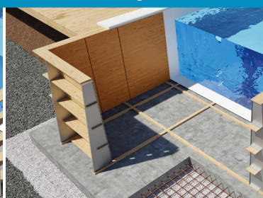
Stomme av trä/betong
