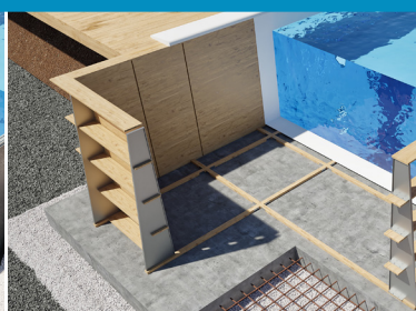
Stomme av trä
