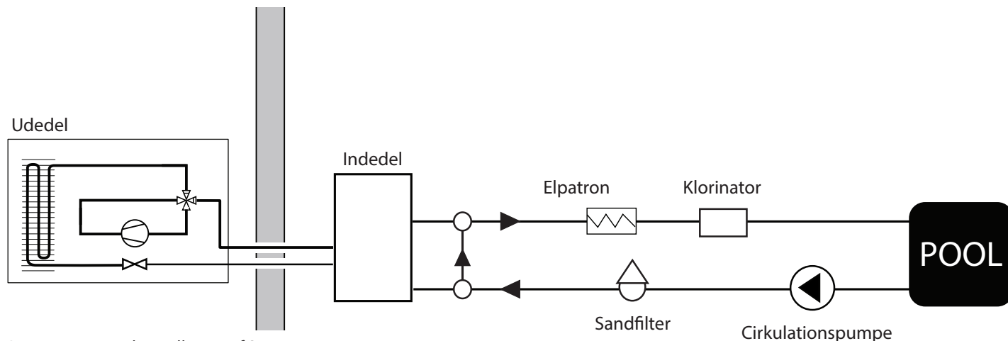
Principtegning til installation af SXX.
