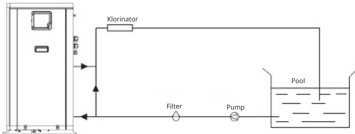
Prinsippskisse for installasjon
